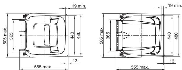
Coperchio standard
