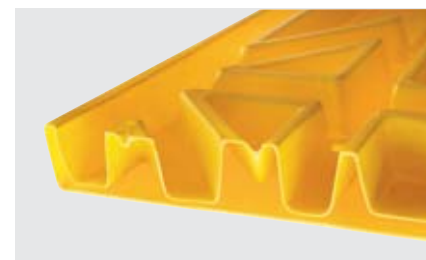
particolare della doppia parete del fondo
